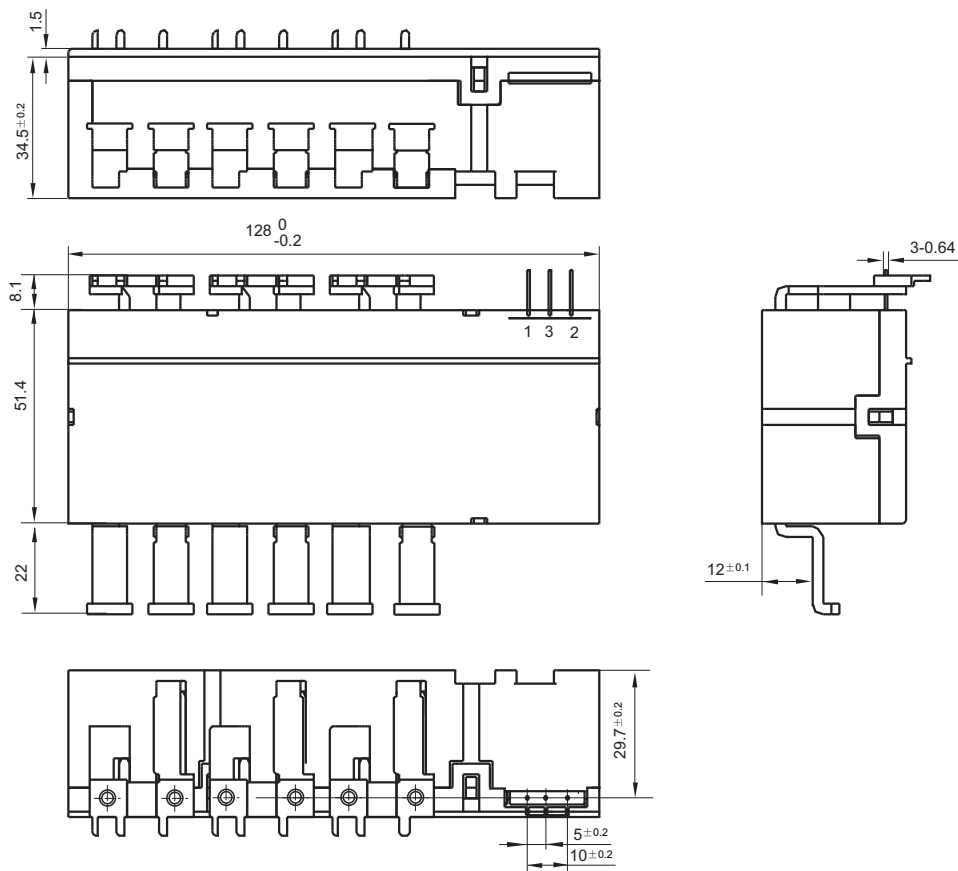
外形图
