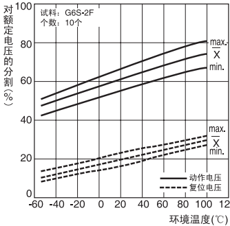
环境温度和动作·复位电压 G6S-2F(G)
