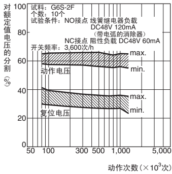
接触可靠性试验*1、*2 G6S-2F(G)
