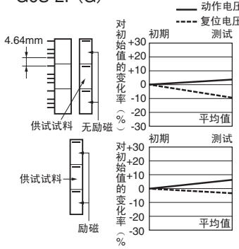
电磁干扰(继电器相互) G6S-2F(G)
