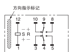
端子配置/内部连接图 (TOP VIEW)
