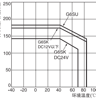
环境温度和最大容许电压 (闭锁型)
