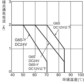
环境温度和接点通电电流 (单稳型)
