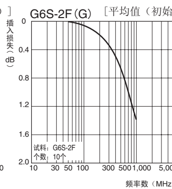
高频特性(插入损失)*1、*3
