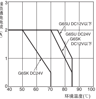
环境温度和接点通电电流 (闭锁型)
