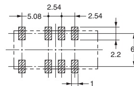
印刷基板加工尺寸 (TOP VIEW) 尺寸公差±0.1mm
