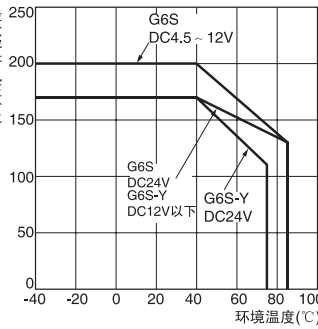
环境温度和最大容许电压 (单稳型)
