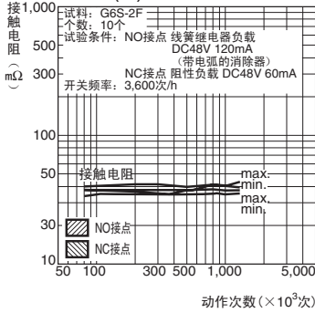
电气的寿命(接触电阻)*1 G6S-2F(G)
