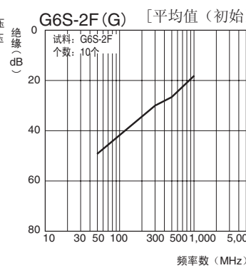
高频特性(绝缘)*1、*3
