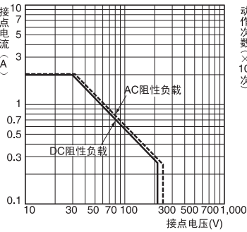
开关容量的最大值
