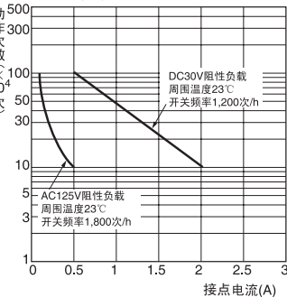
寿命曲线 G6S-2F(G)
