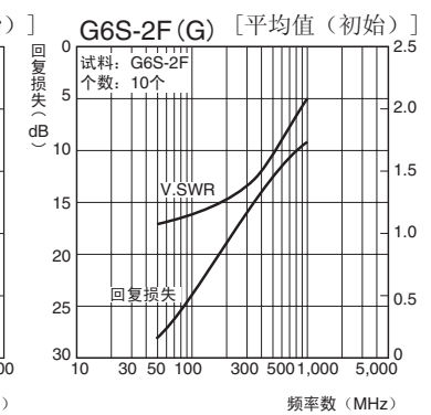
高频特性(回复损失)*1、*3
