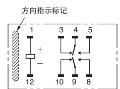
端子配置/内部连接图 (BOTTOM VIEW)
