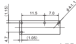
印刷板加工图 (BOTTOM VIEW)
