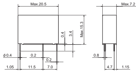
外形尺寸图
