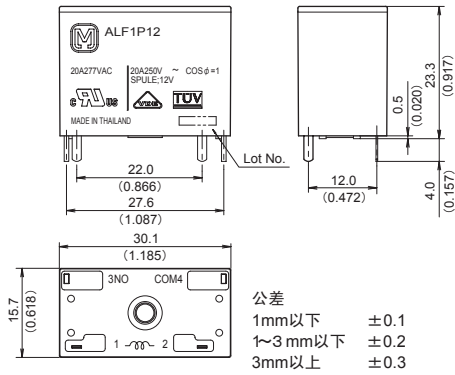
外形尺寸图
