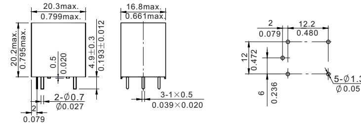
外形尺寸图
