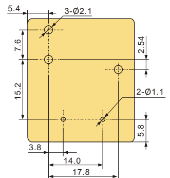
安装孔尺寸图
