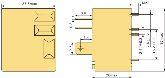
外形图
