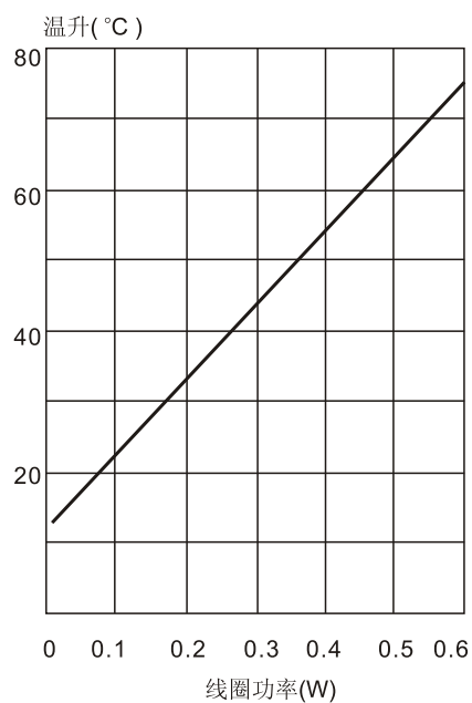
线圈温升
